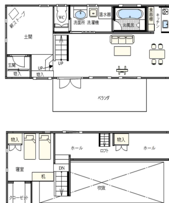
なかとんべつ住宅 間取り図
